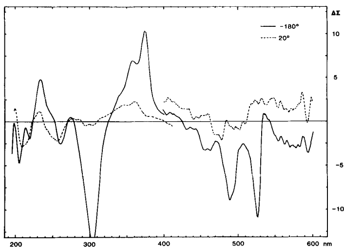
Fig. CD-Spektrum von synthetischen (all-E)-1 in EPA
