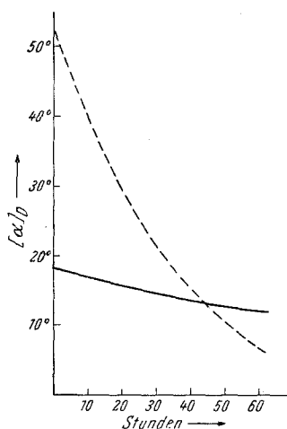
Abb. 1. Drehungsabfall in Äthanol bei 15^{\circ} . — Isopelletierin. - - - Methylisopelletierin.
