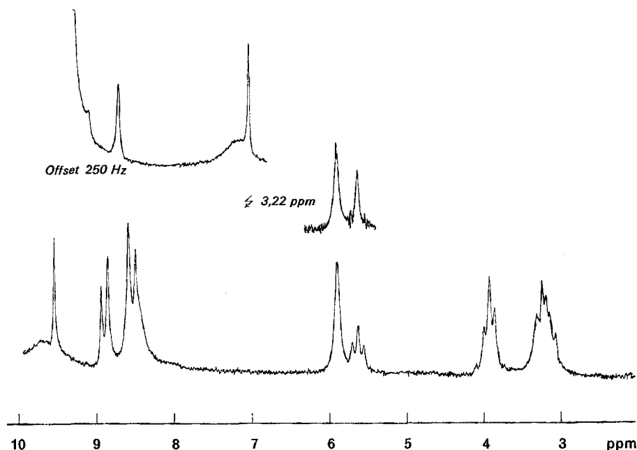
Fig. 3. NMR.-Spektrum (100 MHz) von Folsäure-dihydrat (VI) aufgenommen in \text{FSO}_3\text{H} . Durch Doppelresonanz werden die Signale von \text{C}(\alpha)\text{H} und \text{C}(\beta)\text{H}_2 zugeordnet
