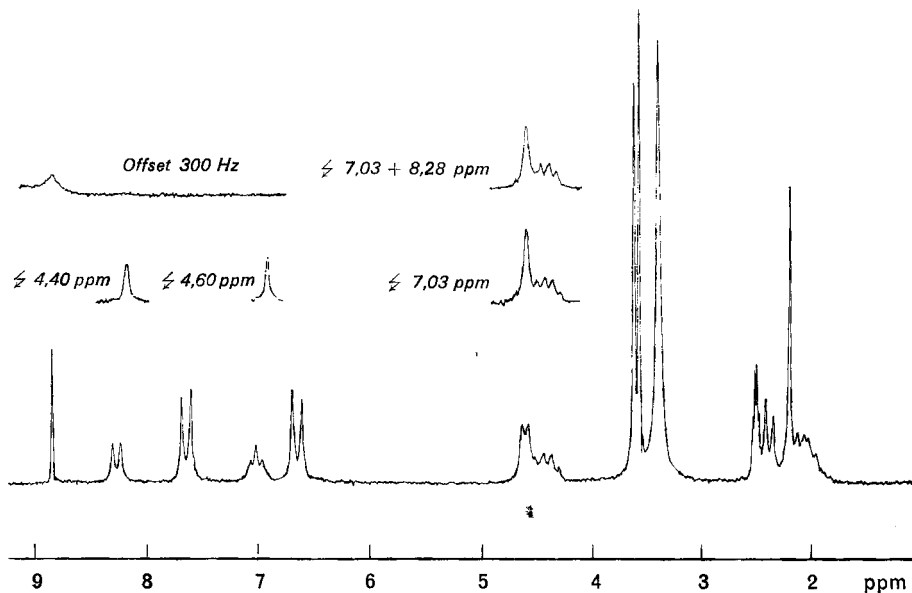
Fig. 2. NMR.-Spektrum (100 MHz) von N (2')-Acetyl-folsäure-dimethylester-dihydrat (V) aufgenommen in d_6 -DMSO. Durch Doppelresonanz werden die Signale von C(9)H 2 und N(10)H bzw. C(α)H und CO(7')-NH zugeordnet
