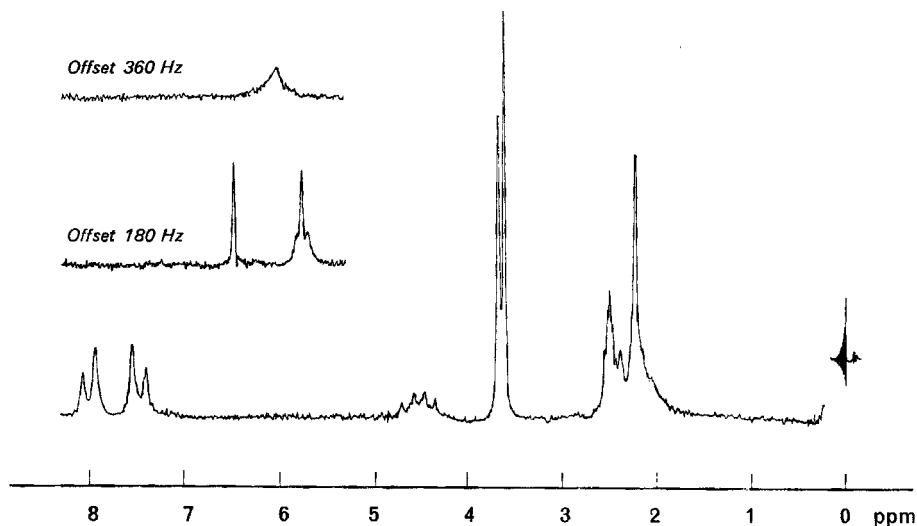
Fig. 1. NMR.-Spektrum (60 MHz) von N (2')-Acetyl-6-[ N -( p -benzoyl- L -glutaminsäure-dimethylester)-azomethin]-pterin (IV) aufgenommen in d_6 -DMSO
