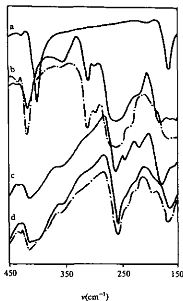
FIG. 8. Far infrared spectra of \text{Co}(\text{bipy})_x\text{Cl}_2 . — solid product; - - - solution product. (a) \text{bipy} ; (b) \text{Co}(\text{bipy})\text{Cl}_2 ; (c) \text{Co}(\text{bipy})_2\text{Cl}_2 ; (d) \text{Co}(\text{bipy})_3\text{Cl}_2 .
