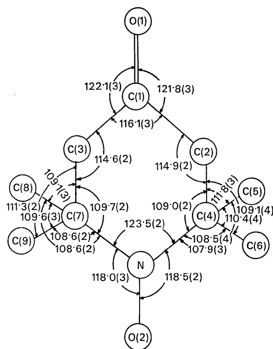
Fig. 1. Distances et angles de la molécule.
