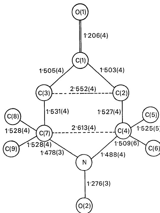
Fig. 1. Distances et angles de la molécule.
