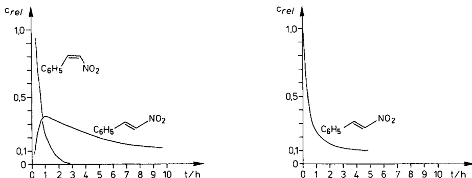
Fig. 2. Abhängigkeit der Konzentrationen von (Z)- und (E)-Nitrostyrol 11 bzw. 9 bei der Umsetzung mit 4-(1-Cyclohexenyl)morpholin von der Zeit. Die Reaktion wurde im NMR-Rohr in (D_{10})Et_2O als Lsgm. verfolgt. Sie führt unabhängig von der Nitrostyrol-Konfiguration zum (u)-Produkt 24 (s. Schema 3).
