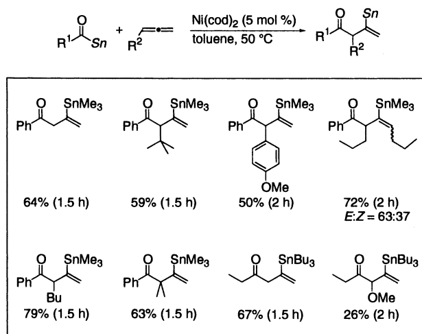
Scheme 18.
