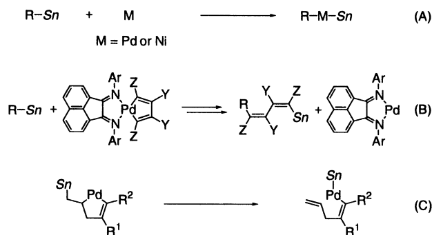
Scheme 20.
