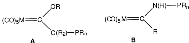
Schema 1. Metallcarbenkomplexe A , B mit Phosphanylgruppen in der Carben–Ligandeneinheit mit unterschiedlich koordiniertem Phosphor.
