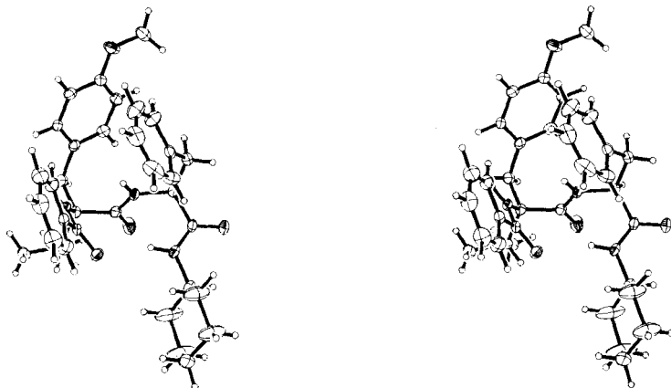
Fig. 1. Stereoplot (ORTEP) of 4b
