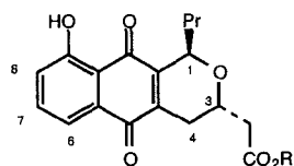
(1 R ,3 S )- 13 R=Me (1 R ,3 S )- 13' R=H
