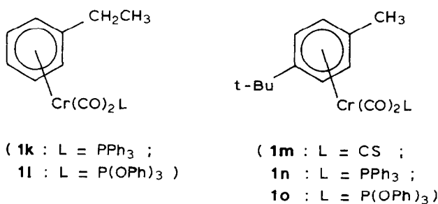
SCHÉMA 1. Complexes ArCr(CO) 2 L.
