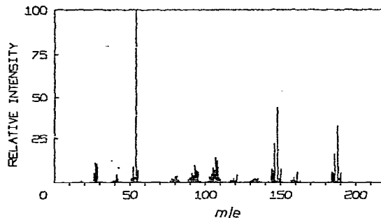
Fig. 3. \text{S}(\text{CH}_2\text{CH}_2\text{CN})_2 .
