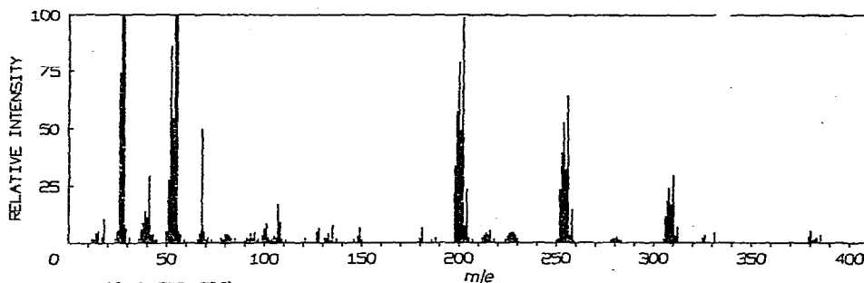
Fig. 1. \text{Hg}(\text{CH}_2\text{CH}_2\text{CN})_2 .
