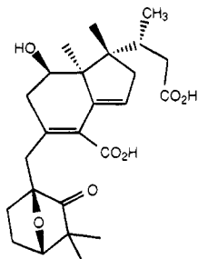
Glycinoeclepin A
