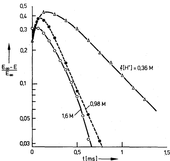
Abb. 2. Auftragung von E_\infty - E/E_\infty gegen die Zeit t nach dem Strahlungspuls in halblogarithm. Maßstab (Daten nach Abb. 1)
