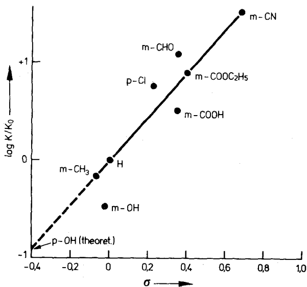
Abb. 6. \log K/K_0 als Funktion der Hammett -Konstanten \sigma für verschiedene Substituenten X am Nitrosobenzolhydrat \text{XC}_6\text{H}_4\text{N}(\text{OH})_2 ( K_0 = Dissoziationskonstante des protonisierten Nitrosobenzolhydrats als Grundkörper)
