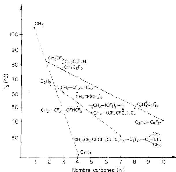
Fig. 1. Variation de la T_g des polymères d'acrylates \text{CH}_2=\text{CH}-\text{C}(\text{O})\text{OR} en fonction du nombre, n , carbones. Les groupements indiqués sont les groupements R de l'acrylate.
