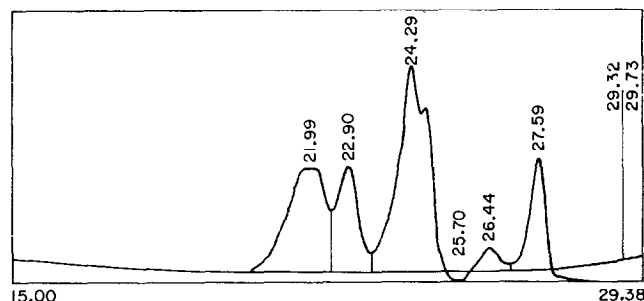
Fig. 2. Chromatogramme GPC de l'homopolymère du N-4-(2'-F-hexyléthoxy)phénylmaléimide.
