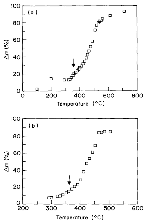
Fig. 5. Thermogrammes \Delta m = f(T) . (a) Pour le copolymère MF I (MF/CEVE=1,1); (b) pour le copolymère MF III (MF/CEVE=2,8).
