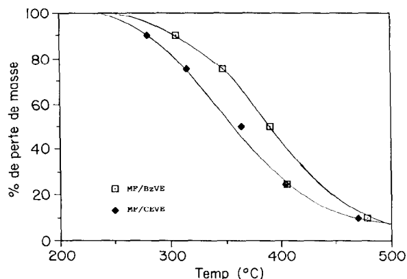
Fig. 4. Thermogrammes sous N_2 des copolymères MF/BzVE et MF/CEVE.
