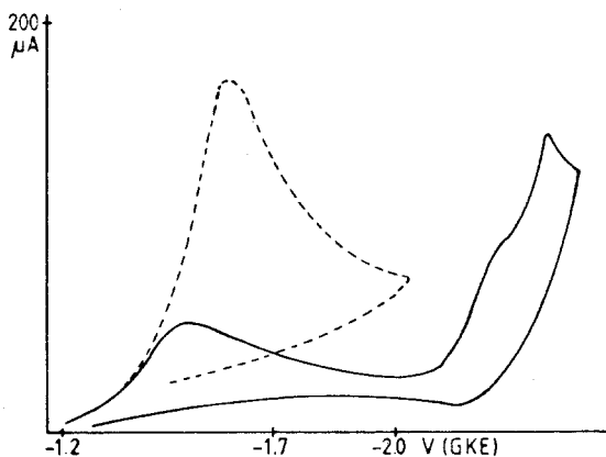
Abb. 1. Reduktion von 10^{-2} M/1 \alpha -Azidostyrol ( 1 ) am hängenden Hg-Tropfen, 100 mV/s, ohne und mit Acetanhydrid
