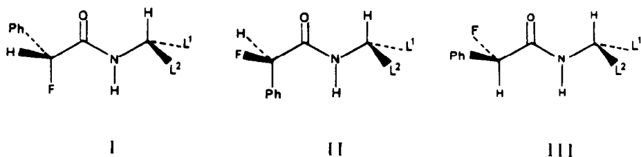
Schéma 1. Conformations des amides PhCHFCONHCHL^1L^2 dans la configuration RR.
