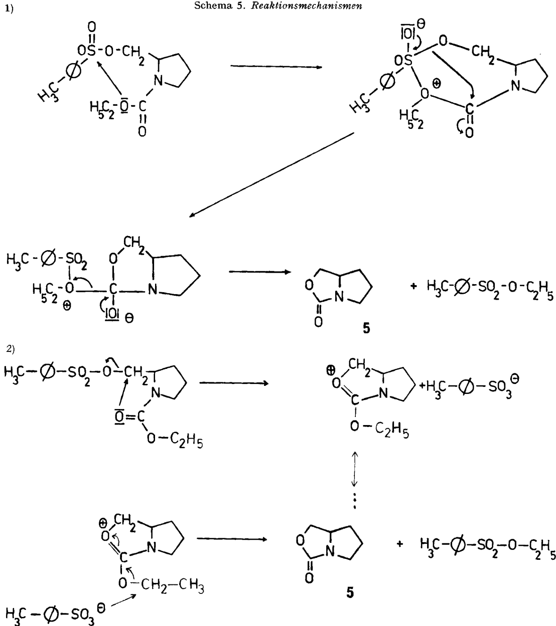
Schema 5. Reaktionsmechanismen
