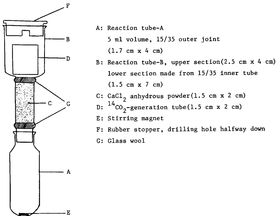
Fig. 1 Apparatus
