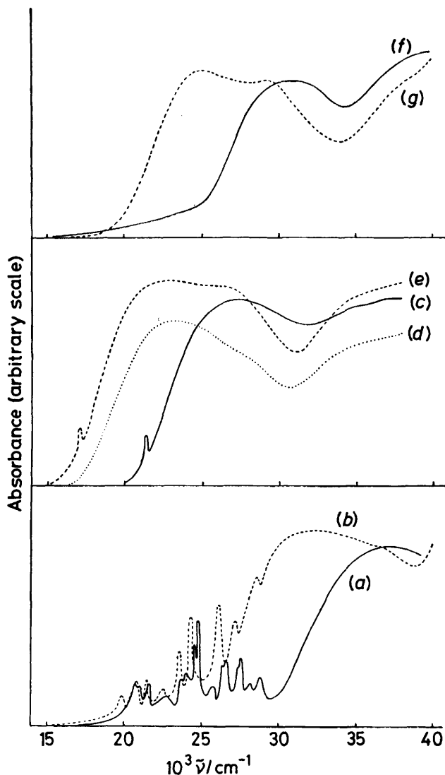
FIGURE 4 Reflectance spectra of the compounds: (a) Sm[ClO _4 ] _3 ·L ^1 ·1.5MeCN·H _2 O; (b) Sm[ClO _4 ] _3 ·L ^3 ·H _2 O; (c) Eu[ClO _4 ] _3 ·L ^1 ·2MeCN·H _2 O; (d) Eu[ClO _4 ] _3 ·L ^2 ·H _2 O; (e) Eu[ClO _4 ] _3 ·L ^3 ·H _2 O; (f) Yb[ClO _4 ] _3 ·L ^1 ·1.5MeCN·H _2 O; (g) Yb[ClO _4 ] _3 ·L ^3 ·H _2 O
