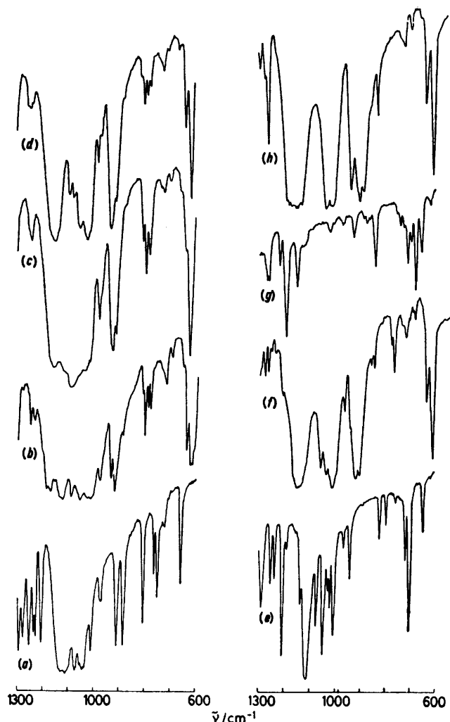
FIGURE 3 Infrared spectra in the 600–1 300 \text{cm}^{-1} region of the compounds: (a) \text{L}^1 ; (b) [\text{La}(\text{ClO}_4)_3(\text{OH}_2)\text{L}^1][\text{ClO}_4] ; (c) \text{Nd}[\text{ClO}_4]_3 \cdot \text{L}^1 \cdot 1.5\text{MeCN} \cdot \text{H}_2\text{O} ; (d) \text{Nd}[\text{ClO}_4]_3 \cdot \text{L}^1 ; (e) \text{L}^2 ; (f) \text{Eu}[\text{ClO}_4]_3 \cdot \text{L}^2 \cdot \text{H}_2\text{O} ; (g) \text{L}^3 ; (h) \text{Eu}[\text{ClO}_4]_3 \cdot \text{L}^3 \cdot \text{H}_2\text{O}
