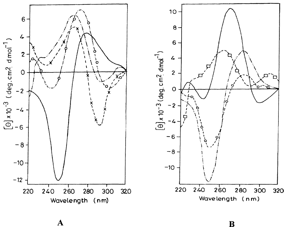
Figure 1. A). CD profiles of 3',5'(C-G) 5 in 1 M NaCl (—), 4 M NaCl (--- × --- × ---) and 2',5'(C-G) 5 in water (---o---o---), 4 M NaCl (· · · · ·). B). CD profiles of 3',5'(G-C) 5 in 1 M NaCl (—), 4 M NaCl (---o---o---) and 2',5'(G-C) 5 in water (—), 4 M NaCl (—□—□—).
