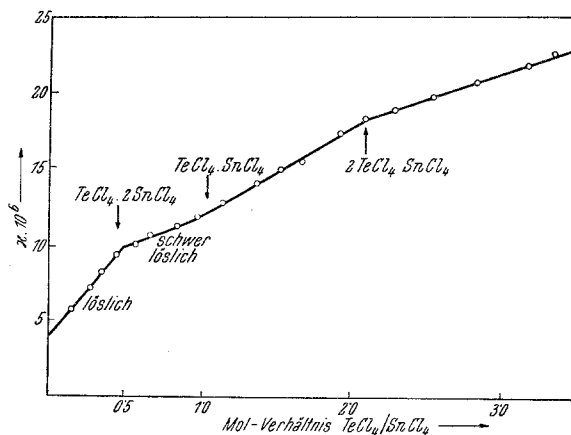
Abb. 2. Leitfähigkeitstiteration in Arsenrichlorid bei 20°. Vorgelegt: 91,5 mg \text{SnCl}_4 in 28 g \text{AsCl}_3 . Titriert mit: Tellurtetrachlorid.
