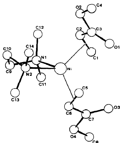
Fig. 1. Kristallstruktur von (tmeda)Ni(H 2 C=CHCOOCH 3 ) 2 (3)
