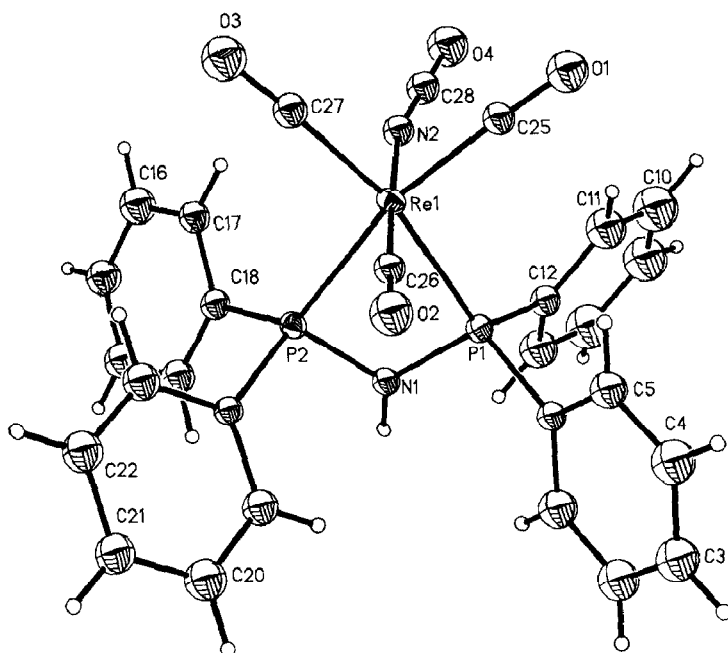
Fig. 3. Struktur von 6b im Kristall.
