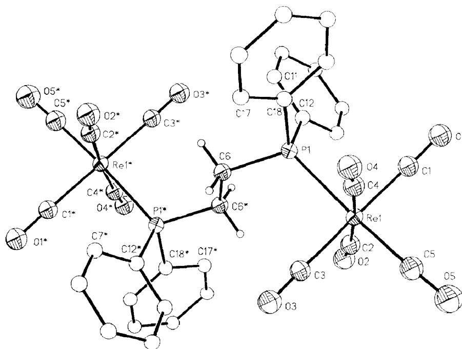
Fig. 2. Struktur von 2c im Kristall.
