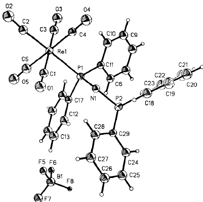
Fig. 1. Struktur von 1a im Kristall.
