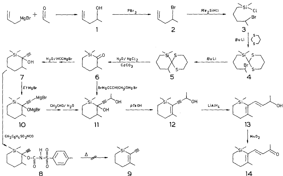
Schema 1. Zur Darstellung von Sila- \beta -Jonon ( 14 ) über 1,1,3-Trimethyl-1-sila-cyclohexan-2-on ( 6 )
