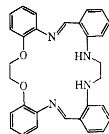
XII, N 4 O 2
