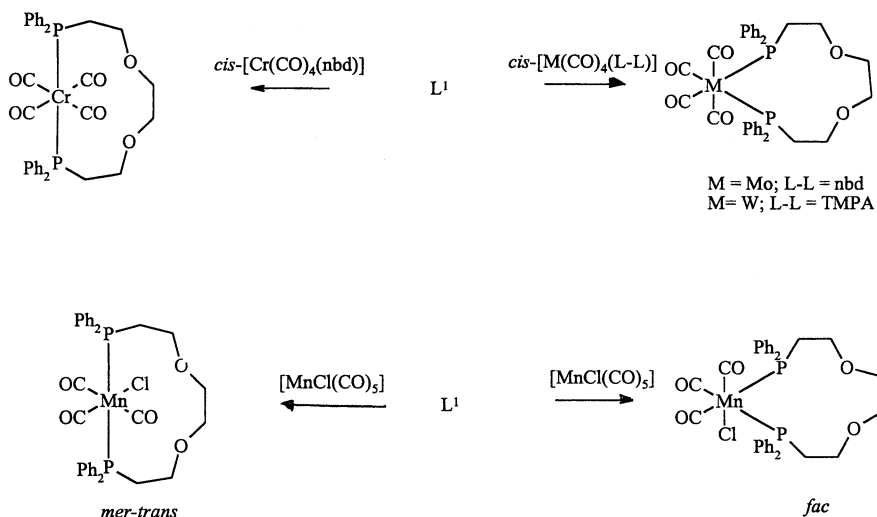
Scheme 1. Complexes of L^1 ( L^1 = Ph_2P(CH_2)_2O(CH_2)_2O(CH_2)_2PPh_2 ).
