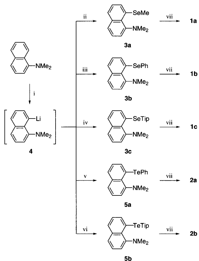
SCHEME 1 Reagents and Conditions: i : BuLi, ether, r.t.; ii : Se powder, then MeI; iii : (PhSe) 2 ; iv : (TipSe) 2 ; v : (PhTe) 2 ; vi : (TipTe) 2 ; vii : Bu t OCl, MeOH, CH 2 Cl 2 , –25°C, then NaOH(aq.)
