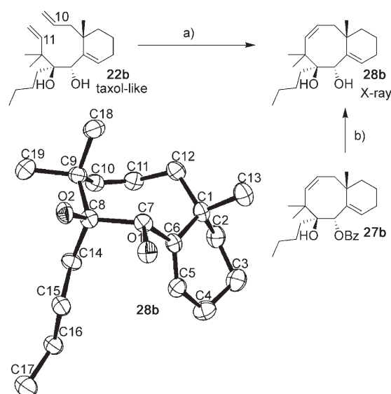
Scheme 10. Metathesis of diol 22b : a) 5 mol % Grubbs 2, CH 2 Cl 2 , reflux, quant.; b) LiAlH 4 , THF, 0 °C, 83 %.
