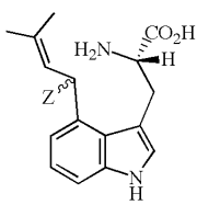
2a (Z = H) 2b (Z = OH)
