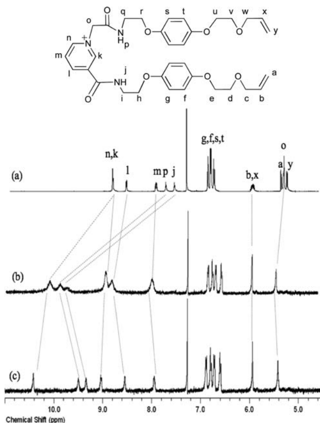
Fig. 1 ^1\text{H} NMR spectra ( \text{CDCl}_3 , 298 K) of (a) \mathbf{6}^+\text{PF}_6^- , (b) (\mathbf{1}^+)_2\text{SO}_4^{2-} and (c) \mathbf{1}^{2+}\text{Cl}^-\text{PF}_6^- .
