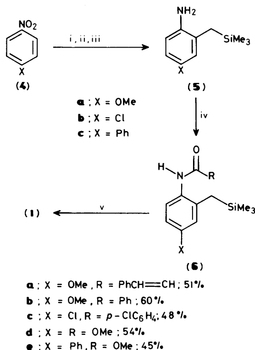
Scheme 2. Reagents and conditions: i, Me 3 SiCH 2 MgCl, THF, 0°C; ii, LiAlH 4 , Pd/C, room temp.; iii, aq. NH 4 Cl; iv, RCOCl, Et 3 N; v, NaH, MeI.
