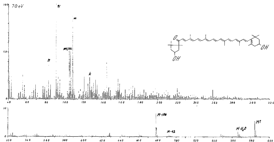
Abb. 19. Massenspektrum von Capsanthin (30)
