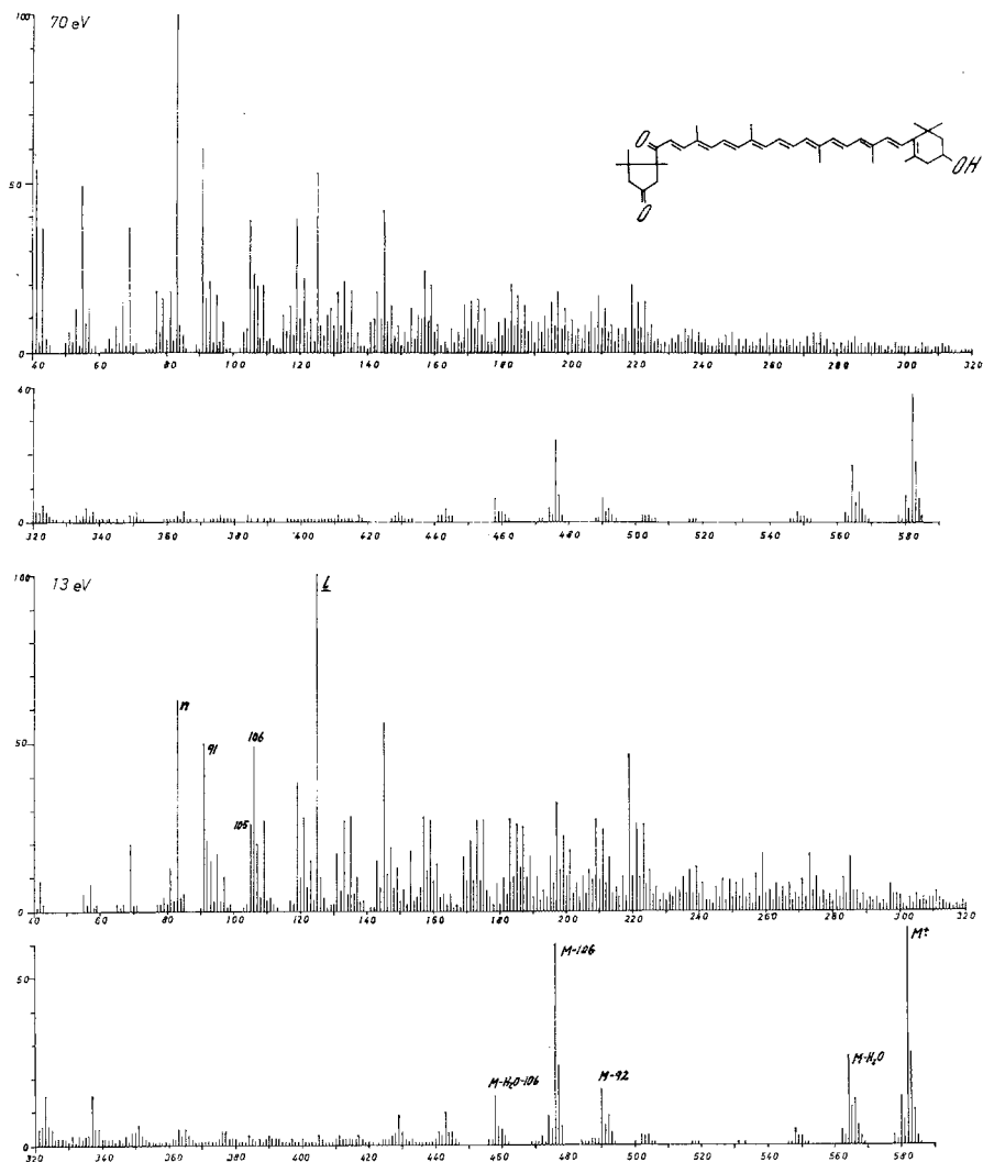
Abb. 20. Massenspektrum von Capsanthon (31)
