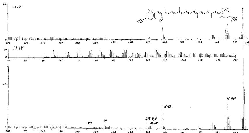
Abb. 3. Massenspektrum von Zeaxanthin-8-d (6). Das 70-eV-Spektrum zwischen m/e 60 und 300 ist uncharakteristisch (vgl. Abb. 1)
