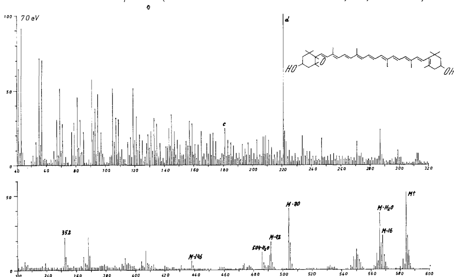
Abb. 7. Massenspektrum von Anthraxanthin ( 14 )
