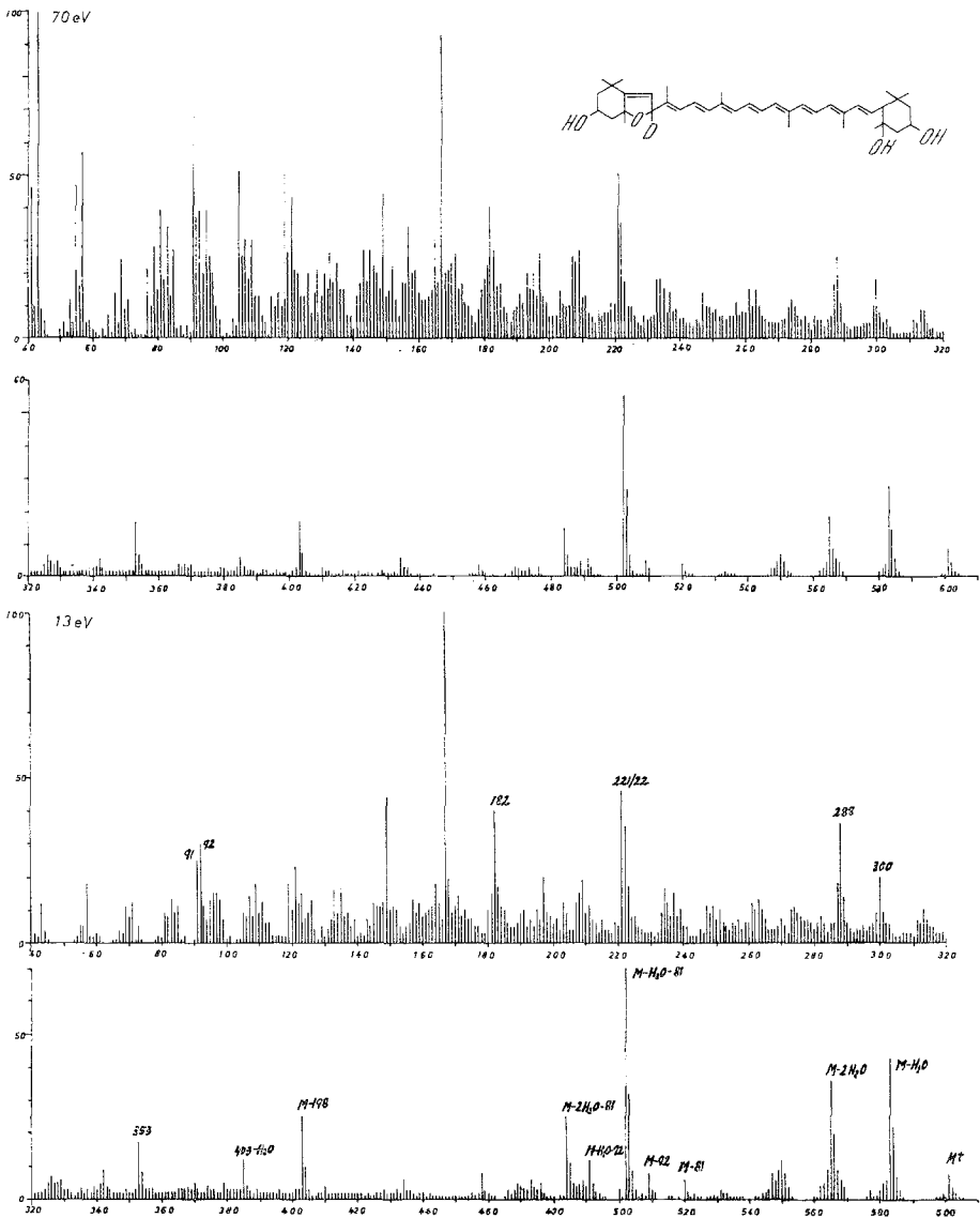
Abb. 12. Massenspektrum von Fucochrom-8-d (19). Anm. bei der Korrektur: In der Formel fehlt die allenische Doppelbindung (vergl. Formel in Abb. 11)
