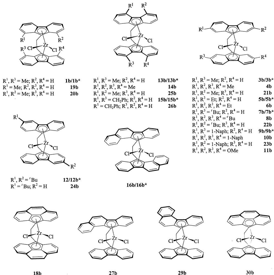
Abb. 3. Übersicht der dargestellten ansa -Bis(fluorenyliden)zirconiumdichloridkomplexe.
