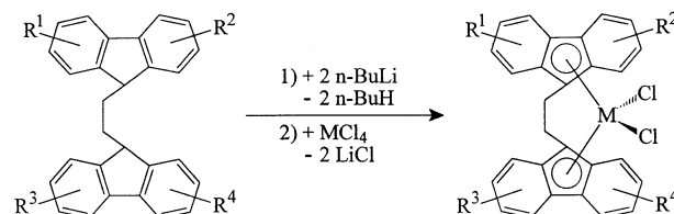
Schema 3. Darstellung der Metallocenkomplexe.
