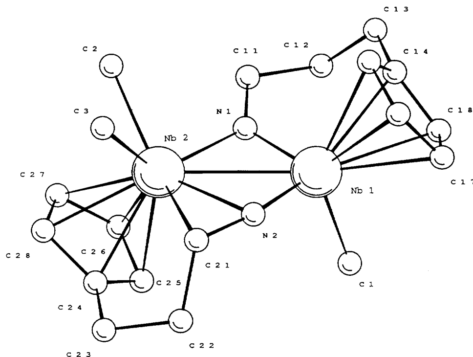
Fig. 1. Molecular structure of \{\text{MeNb}[\eta\text{-C}_5\text{H}_4(\text{CH}_2)_3(\mu\text{-N})(\mu\text{-}\sigma(\text{N})\text{-}\eta^2(\text{N,C})\text{-NCH}(\text{CH}_2)_2\text{-}\eta\text{-C}_5\text{H}_4)]\text{NbMe}_2\} 11 . Hydrogen atoms are omitted for clarity. Selected bond lengths (Å) and angles (deg) as follows: Nb(1)–C(1) 2.21(1), Nb(1)–N(1) 1.901(8), Nb(1)–N(2) 1.847(8), Nb(1)–Nb(2) 2.929(1), Nb(2)–C(2) 2.26(1), Nb(2)–C(3) 2.28(1), Nb(2)–N(1) 2.134(7), Nb(2)–N(2) 2.225(7), Nb(2)–C(21) 2.32(1), N(2)–C(21) 1.34(1), C(21)–C(22) 1.55(2); Nb(1)–N(1)–Nb(2) 92.9(3), Nb(1)–N(2)–Nb(2) 91.5(3), C(21)–N(2)–Nb(1) 168.0(7), C(21)–N(2)–Nb(2) 76.6(5), C(11)–N(1)–Nb(2) 133.0(6), C(11)–N(1)–Nb(1) 133.7(6), C(14)–C(13)–C(12) 114.9(9), C(12)–C(11)–N(1) 114.6(9), N(2)–C(21)–Nb(2) 69.1(5), C(22)–C(21)–N(2) 118.0(9), C(22)–C(21)–Nb(2) 116.0(8), C(23)–C(22)–C(21) 107.9(9), C(24)–C(23)–C(22) 107.9(8).
