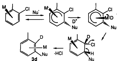
Schéma 2. Pour simplifier, l'entité Cr(CO) _3 a été représentée par M.
