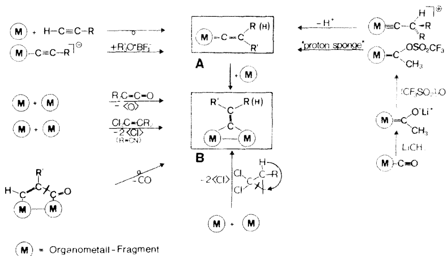
SCHEMA 1. Gebräuchliche Darstellungsverfahren für Vinyliden-Komplexe
