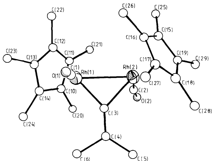
Fig. 1. Molekülstruktur von \mu -Dimethylvinyliden-bis[carbonyl( \eta^5 -pentamethylcyclopentadienyl)rhodium]-(Rh–Rh) ( 3a ) im Kristall. Die Wasserstoffatome wurden bei der Strukturbestimmung nicht lokalisiert und sind daher auch in der Zeichnung weggelassen.
