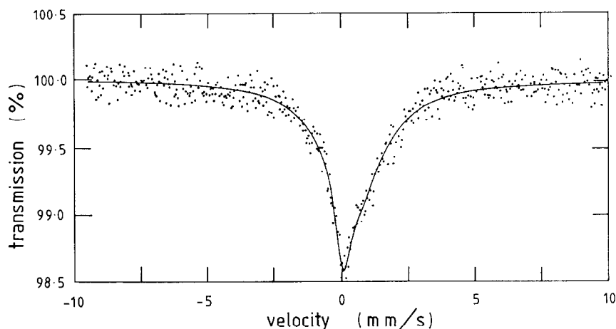
Fig. 1. ^{57}\text{Fe} Mössbauer spectra of [T(MeO) _3 PPFeCl] at 78 K.
