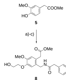
Scheme 2. Synthesis of the linker group 8 . a) THP-OCH 2 CH 2 Br, K 2 CO 3 , DMF, 90 °C, 10 h, 94 % ( \rightarrow 6 ); b) PhCH 2 C(O)NHCH 2 OH, HOAc/H 2 SO 4 20:1, 20 °C, 10 h, 83 % ( \rightarrow 7 ); c) NaOMe, MeOH, 0 °C, 1 h, 87 %.
