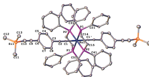
Fig. 2 Molecular structure of 3a . Selected bond lengths (Å) and angles (°): Ru(1)–P(1), 2.3598(6), 2.3555(7); Ru(1)–C(1), 2.066(3); C(1)–C(2), 1.204(4); C(2)–C(3), 1.438(4); C(6)–C(9), 1.449(4); C(9)–C(10), 1.197 (4); C(10)–Si(1), 1.836(3); P(1)–Ru(1)–P(1') 180.0.
