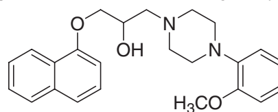
Naftopidil
