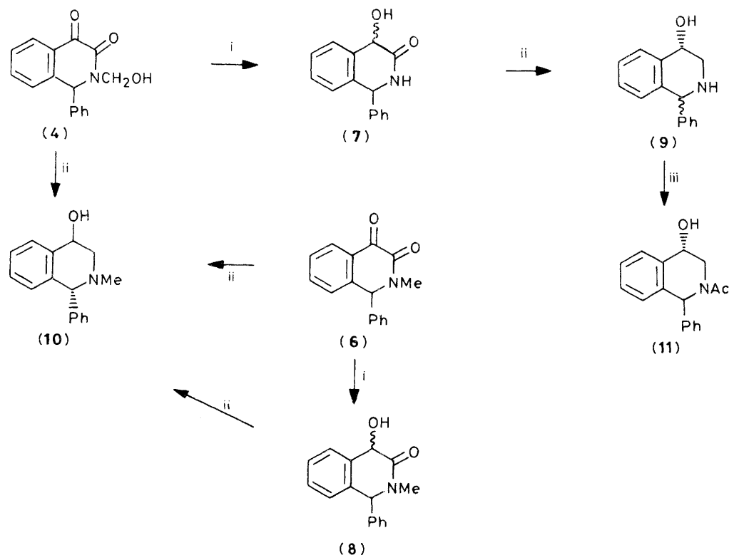
Scheme 2. Reagents: i, \text{NaBH}_4 ; ii, \text{LiAlH}_4 ; iii, \text{Ac}_2\text{O} , \text{AcOH}
