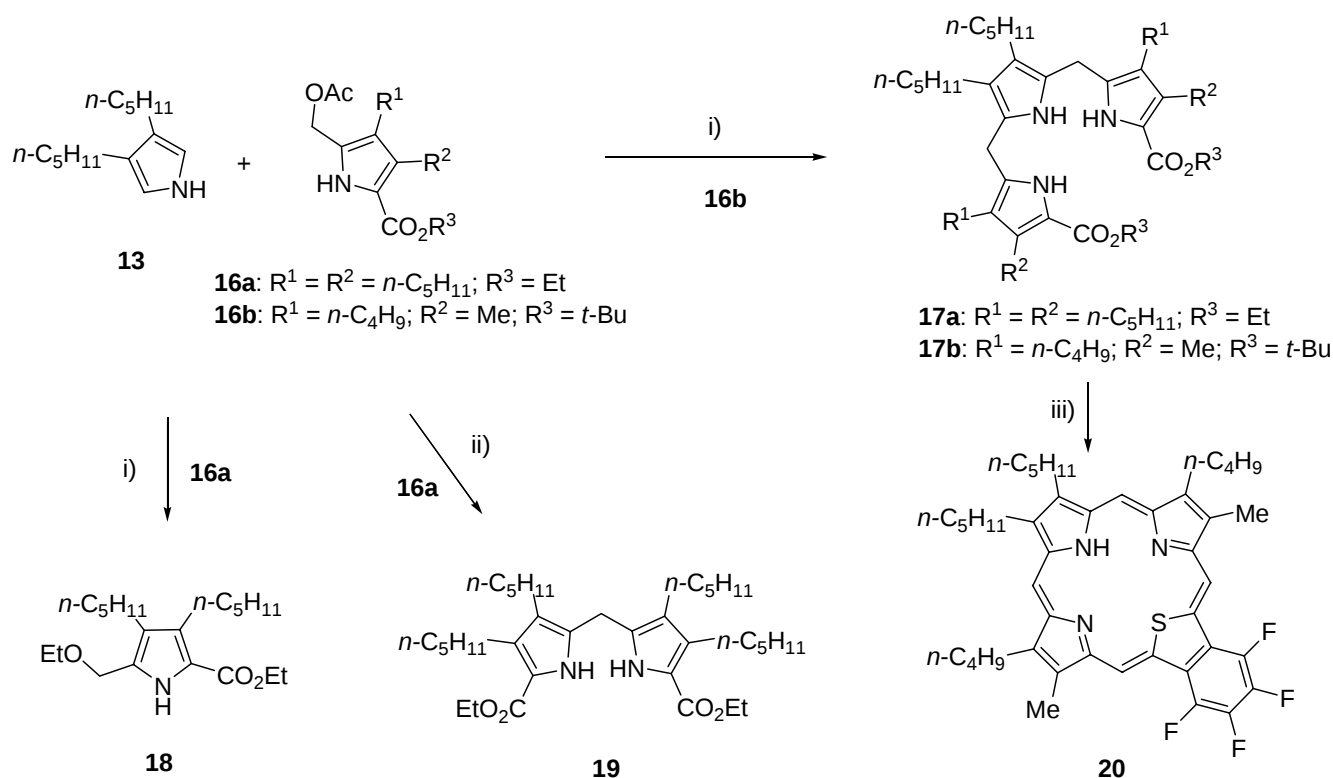
Scheme 4. Reagents and conditions: i) AcOH/EtOH, reflux. ii) AcOH/ \text{CF}_3\text{CH}_2\text{OH} , reflux. iii) 9 , TFA, \text{CH}_2\text{Cl}_2 , rt; \text{Et}_3\text{N} ; DDQ.
