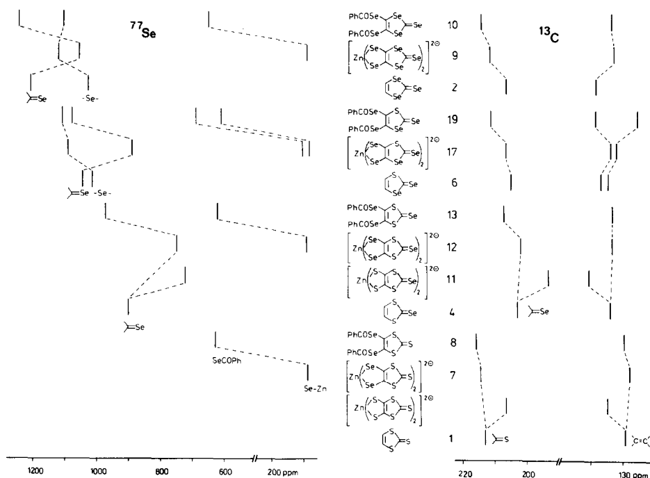
Fig. 1. ^{77}\text{Se} - und ^{13}\text{C} -NMR-chemische Verschiebungen der untersuchten Verbindungen.
