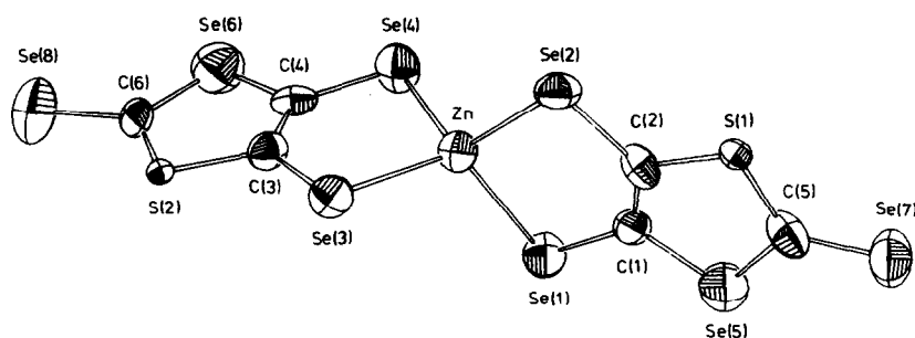
Fig. 2. Molekülstruktur des Anions von 18 mit der in Tab. 2 und 3 benutzten Atomnummerierung.
