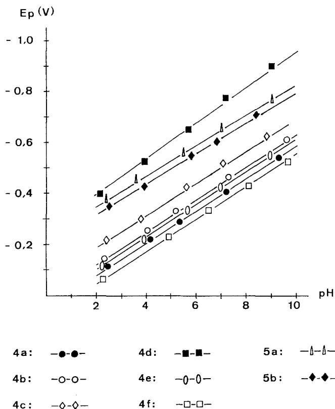
Abb. 2. pH -Abhängigkeit der Peakpotentiale der Isoindoldionderivate 4a–f und 5a–b in BRP ( 4d : 10% DMF, 4f : 30% EtOH, alle übrigen 10% EtOH)
