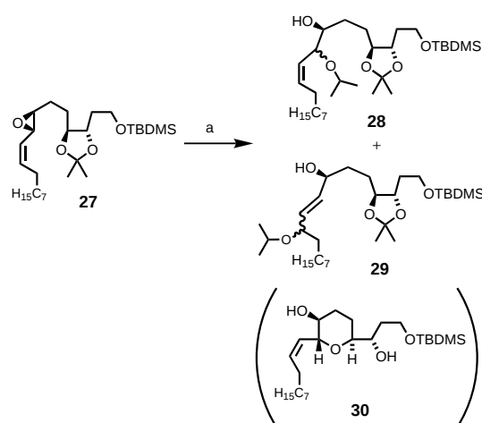
Scheme 5. a) CSA (8 mol %), \text{CH}_2\text{Cl}_2/i\text{PrOH} (30:1), -60 \rightarrow 20^\circ\text{C} , 16 h, 28 : 13%, 29 : 23%.
