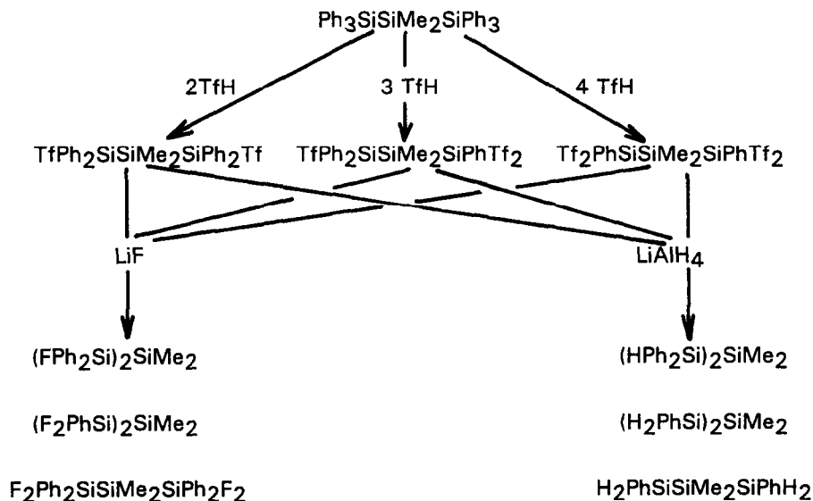
Schema 1. Aus (Ph_3Si)_2SiMe_2 synthetisierte Trisilane.
