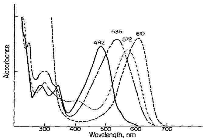
Fig. 1. Absorption spectra of 4-[ p -dimesitylborylphenylazo]-1-naphthol; (—) methanol, \epsilon 29 000; (---) methanol/NaOH, \epsilon 31 400; (· · · · ·) methanol/HCl, \epsilon 28 000; (- · - · -) acetone/NaOH, \epsilon 32 000.
