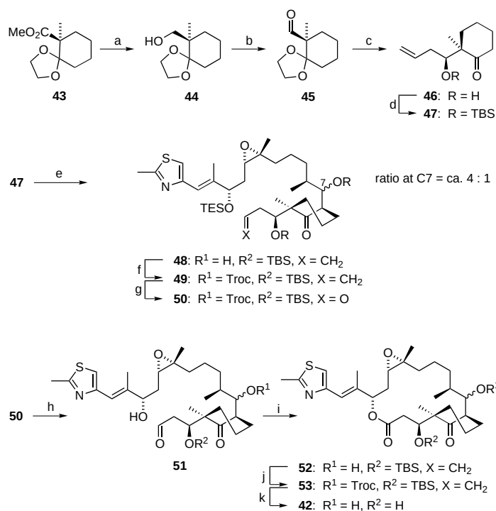
Scheme 5. a) LAH, Et 2 O, 25 °C, 3 h, 97 %; b) oxalylchloride, DMSO, CH 2 Cl 2 , –78 °C, 15 min, then NEt 3 /Pr, 0 °C, 1 h, 90 %; c) (–)-IpcB(allyl), allylmagnesium bromide, Et 2 O, THF, –78 °C, 3 h, workup with H 2 O 2 , NaOH, ds = 6:1, 50 %; d) TBSOTf, 2,6-lutidine, CH 2 Cl 2 , 96 %; e) LDA, THF, –78 °C, 10 min, then 7 , –78 °C, 10 min, 78 %; f) TrocCl, pyridine, CH 2 Cl 2 , 25 °C, 40 min, 98 %; g) OsO 4 , NMO, t BuOH, THF, 25 °C, 16 h, then NaIO 4 , H 2 O, EtOH, 25 °C, 1 h, 64 %; h) HF, pyridine, THF, 25 °C, 20 min, 88 %; i) NaClO 2 , butanol, 2,3-dimethyl-but-2-ene, H 2 O, NaH 2 PO 4 , 25 °C, 2 h, then 2,4,6-trichlorobenzoyl chloride, NEt 3 , toluene, DMAP, 25 °C, 30 min, 36 %; j) Zn, EtOH, NH 4 Cl, reflux, 30 min, 95 %; k) HF, pyridine, 40 °C, 4 d, 50 %. Ipc = isopinocampheyl; LDA = lithium diisopropylamide.
