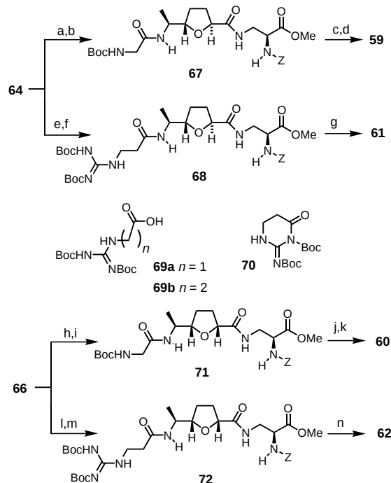
Scheme 9. Synthesis of the RGD-mimetics 59 , 60 , 61 , and 62 : a) TFA, CH 2 Cl 2 , rt, 2 h; b) N -Boc-glycine, HOBT, EDC, EtN( i Pr) 2 , THF, rt, 18 h, 94 % from 64 ; c) i) TFA, CH 2 Cl 2 , rt, 2 h; ii) 54 , HgCl 2 , Et 3 N, DMF, rt, 2.5 h, 93 %; d) i) LiOH, THF, H 2 O, rt, 20 min; ii) TFA, CH 2 Cl 2 , rt, 2 h, 60 %; e) TFA, CH 2 Cl 2 , rt, 2 h; f) 69b , HOBT, EDC, EtN( i Pr) 2 , THF, 0 °C → rt, 3 h, rt, 3 h, 75 % from 64 ; g) see d), 72 %; h) and i): see a) and b), 81 %; j) and k): see c) and d), 67 %; l) and m): see e) and f) 35 % 72 and 29 % 70 ; n) see d), 79 %.
